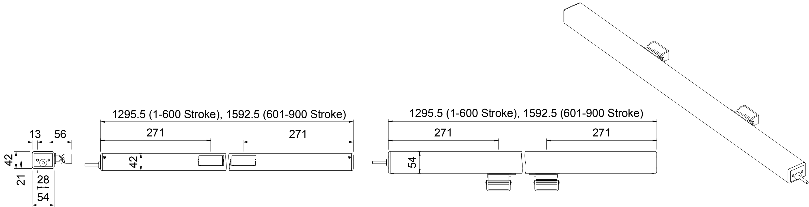
02 SideView 1 : 5
